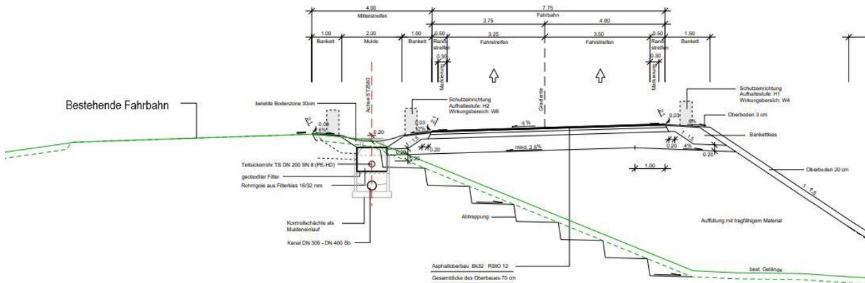
Straßenquerschnitt St 2580 RQ 21 - Bk32 Deckschicht gemäß Anforderungen RLS-90 mit 2 dB (A) Abzug Bau-km 0+000 bis Bau-km 1+300 Bau-km 3+700 bis Bau-km 5+565
